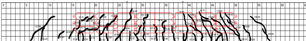
Fig 10 c). Pola retak Balok Uji BR3B
